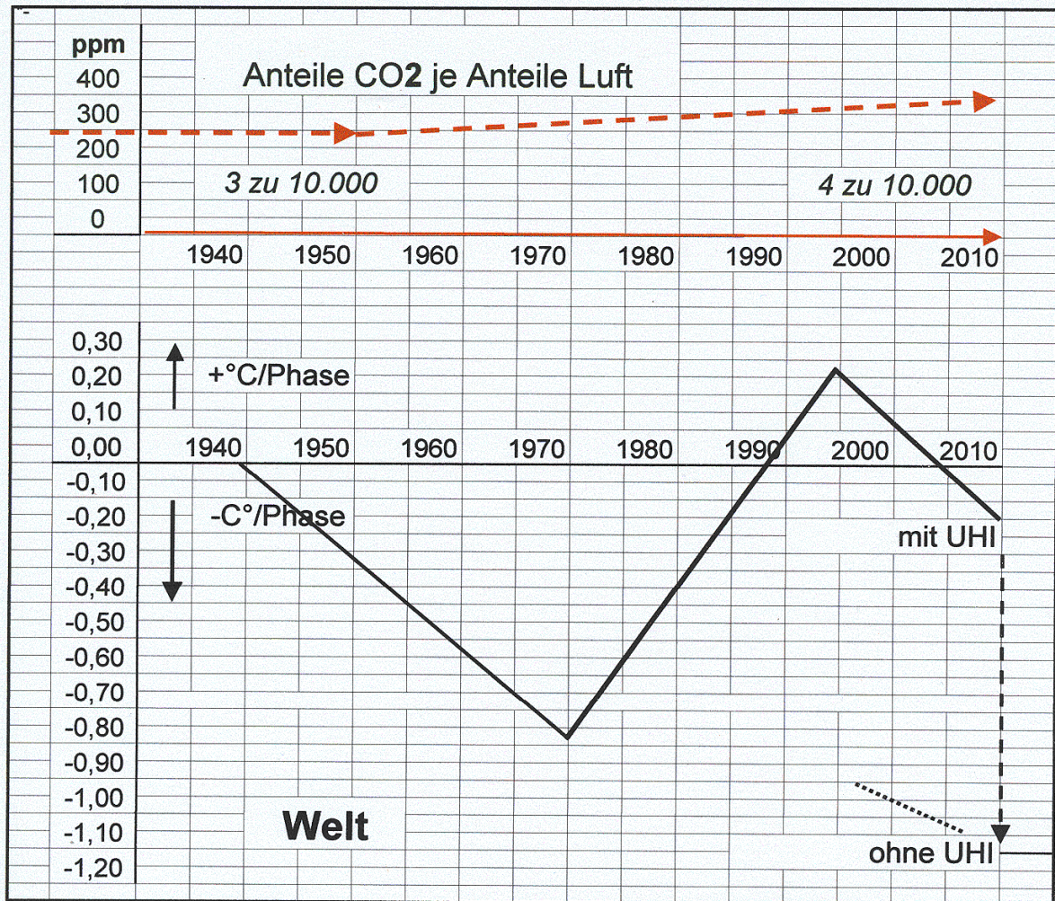
Abb. 13: oben – Zunahme des CO 2 -Anteiles infolge Emissionen; unten – durchschnittliche Trendlinien der Phasen 5, 6 und 7 ergeben mittlere Ganglinie für die Temperaturentwicklung einschließlich UHI-Anteil der Welt für die Zeit 1940 bis 2010, Abzug des UHI-Anteils ergibt naturgegebene Temperatur – gestrichelte Pfeillinie.
