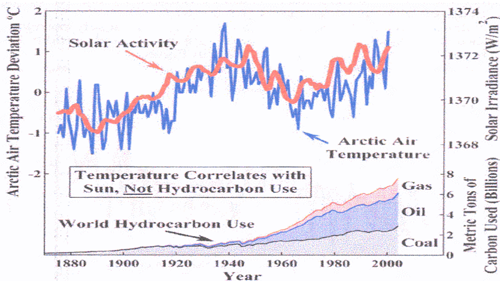
Abb. 4: Einstrahlung, arktische Temperaturen, Förderung von Kohle, Öl und Gas
