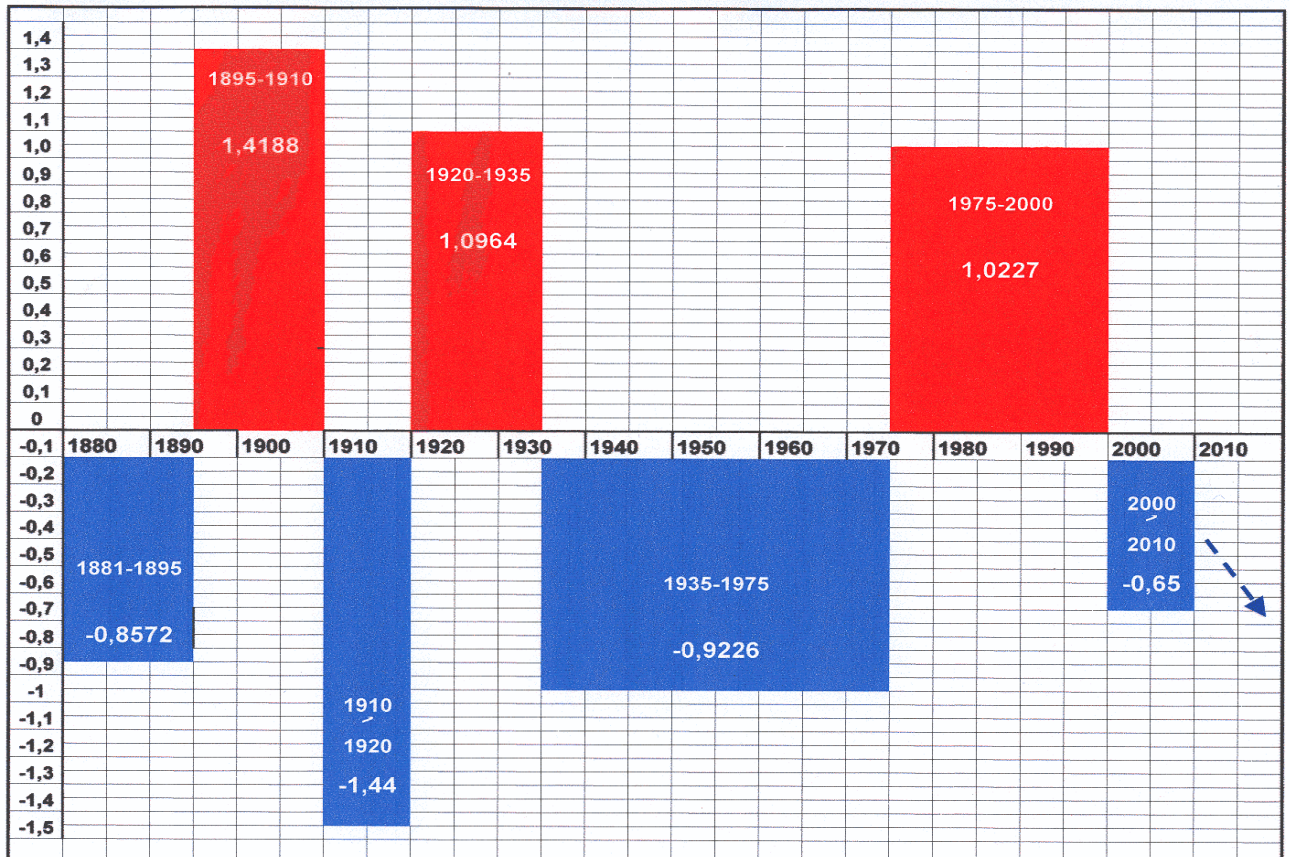
Abb. 11: Mittelwerte für die Dauer der Phasen 1 bis 7 und ihrer Änderungen
